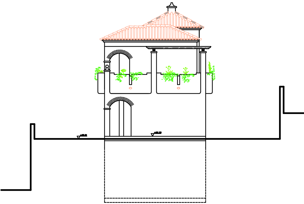
Alzado Lateral Derecho
